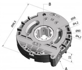
Cardan Mechanism Kg SINFIN R5.3:1 C8 HEX 7 HEX16 SIN FIN FIN
