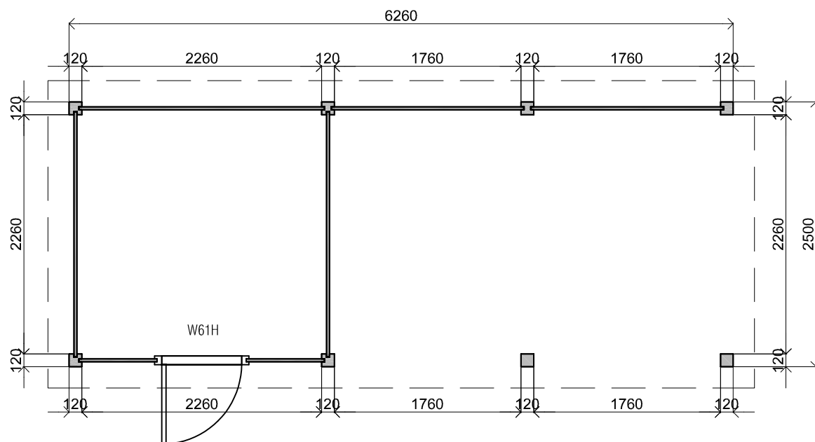
Plattegrond / Plan
