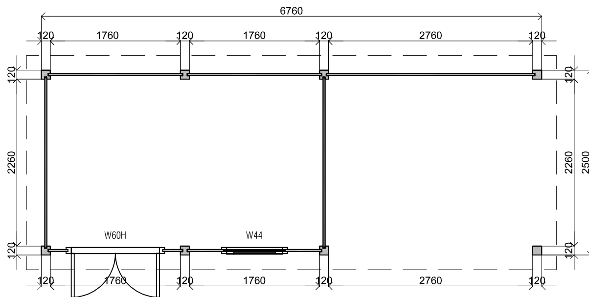
Plattegrond / Plan
