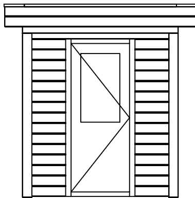
Vooraanzicht / Front view / Vorderansicht
