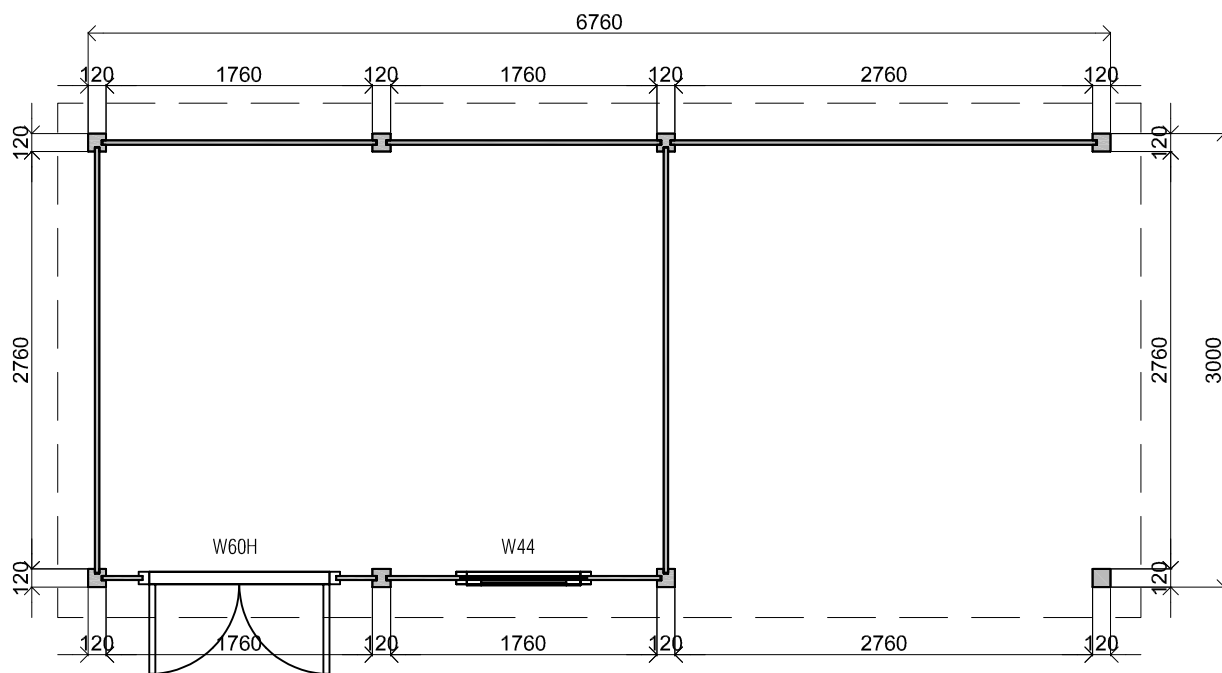
Plattegrond / Plan
