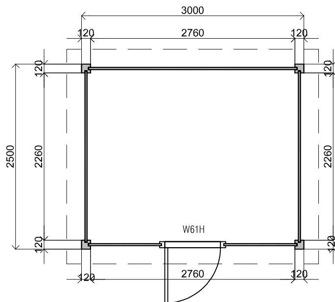
Plattegrond / Plan
