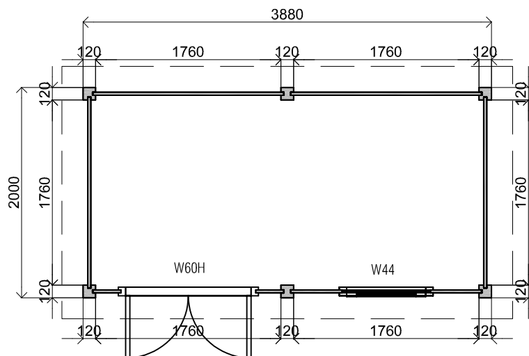
Plattegrond / Plan
