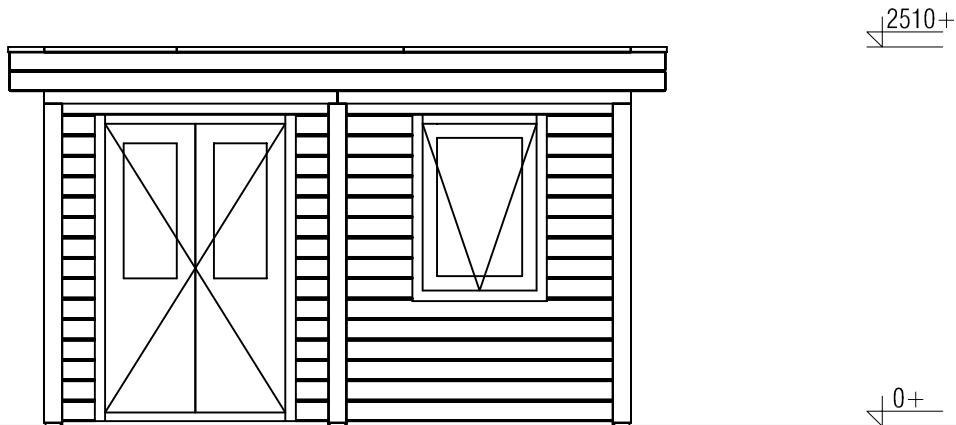
Vooraanzicht / Front view / Vorderansicht
