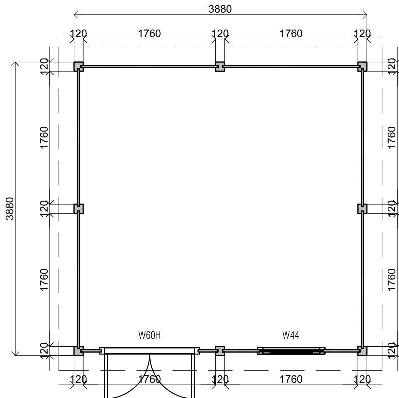
Plattegrond / Plan
